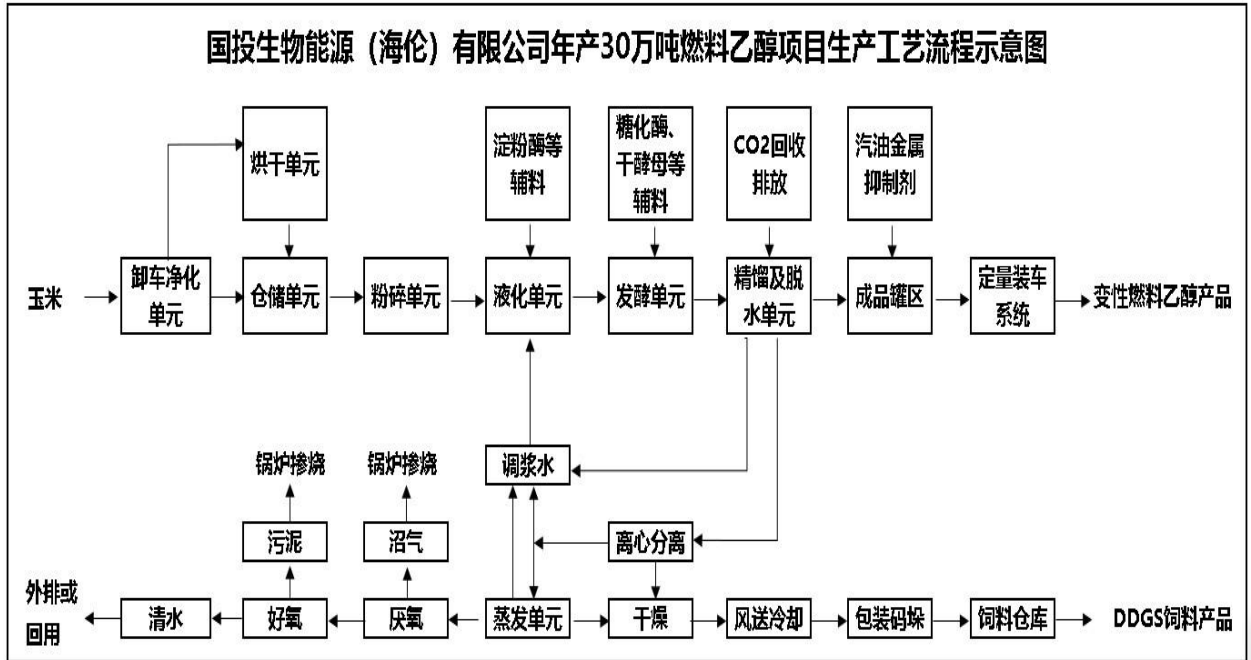
图 1-2 生产工艺流程图
